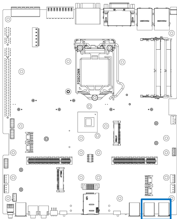
USB3_3, USB3_4
