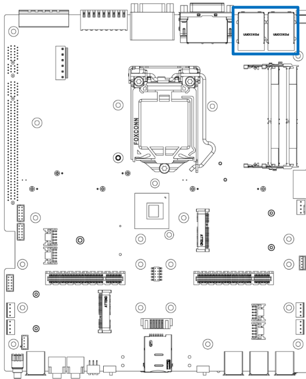
LAN1 LAN2 USB3.1 GEN 4 Ports
