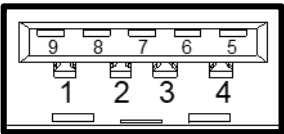
USB3_1, USB3_2
