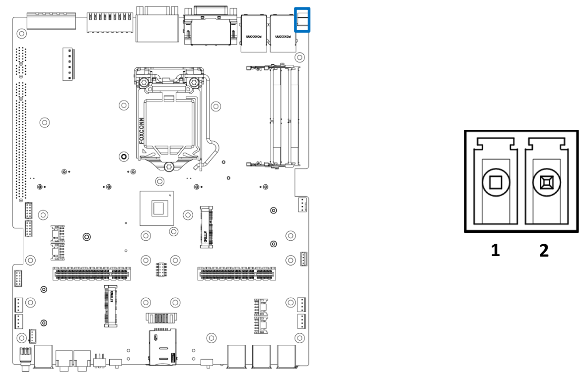
PWRBTN2
