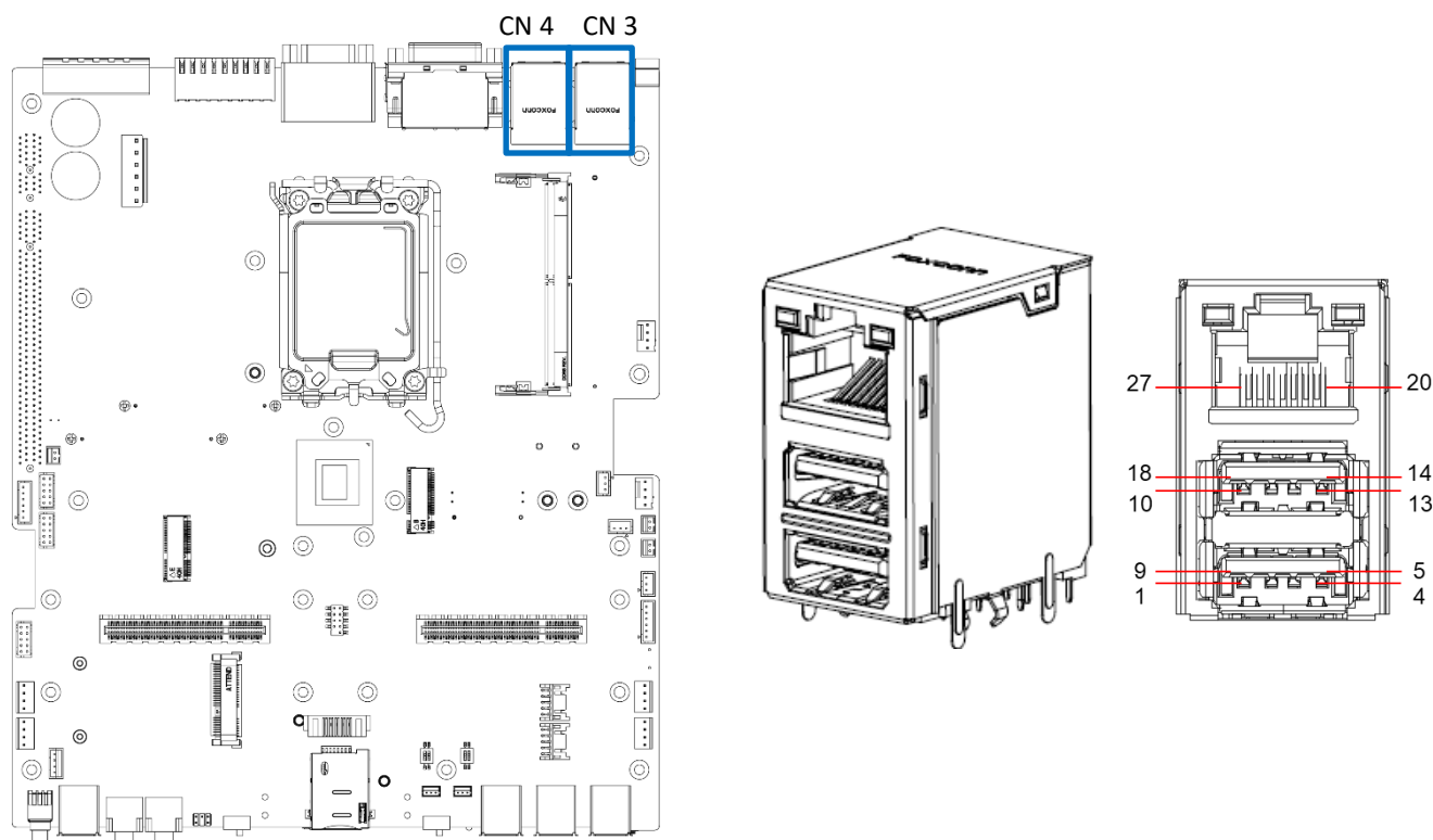
CN3, CN4
