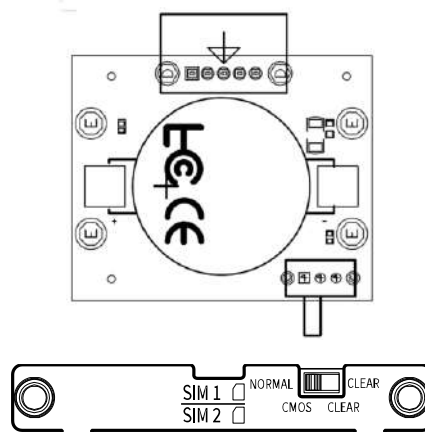
CLR_CMOS
