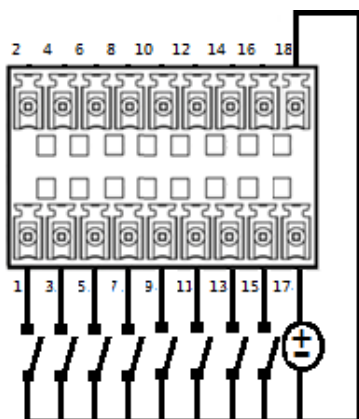
Digital Input Wurung
