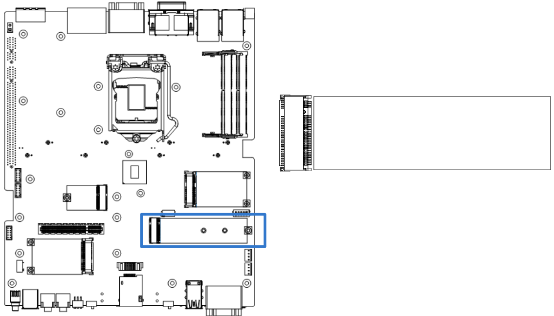
CN2 : M.2 M Key Socket
