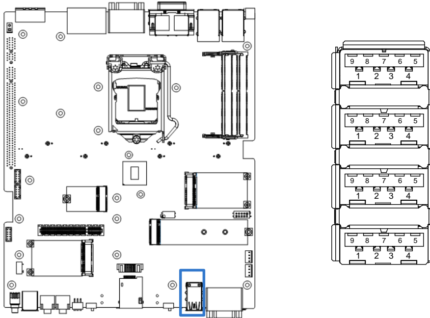
CN6 : USB3.1 Connector, Type A x 4
